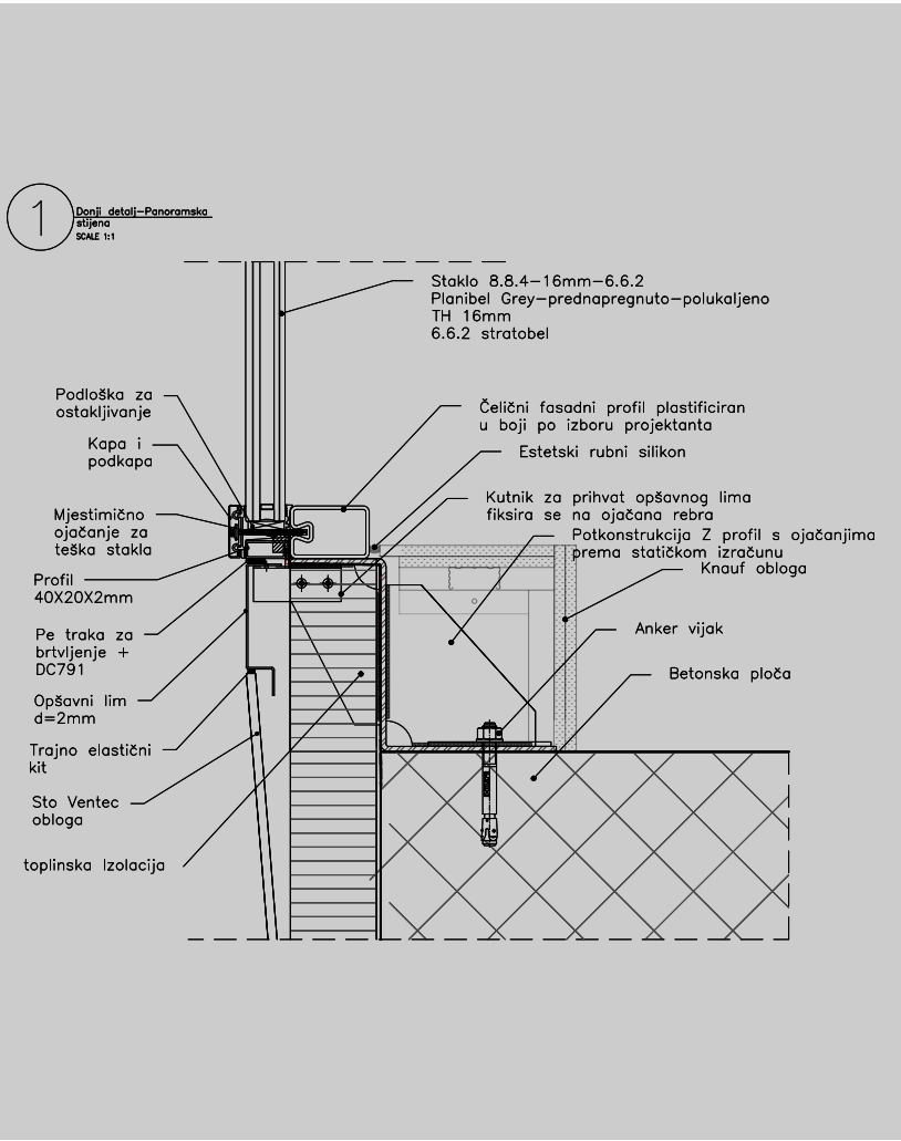
IZVEDBENI DETALJ (Aluk tim)
