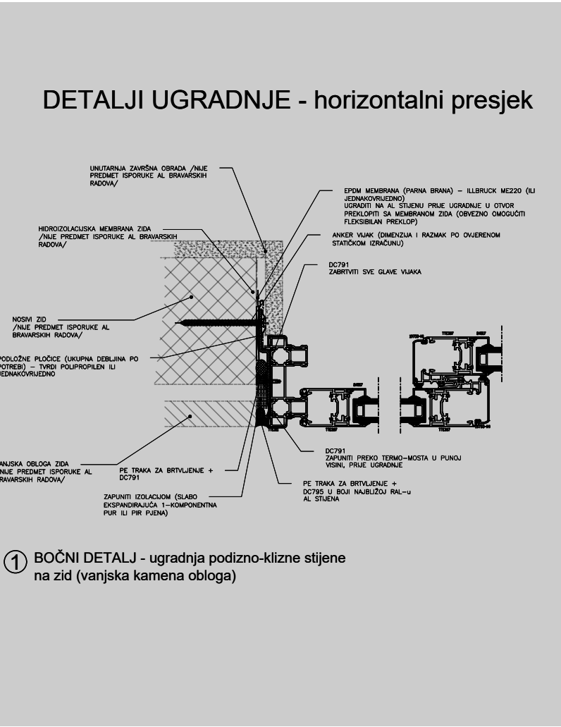
IZVEDBENI DETALJ (Aluk tim)
